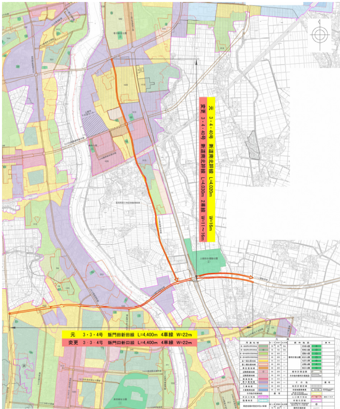
上越都市計画道路の変更（新潟県決定）総括図
